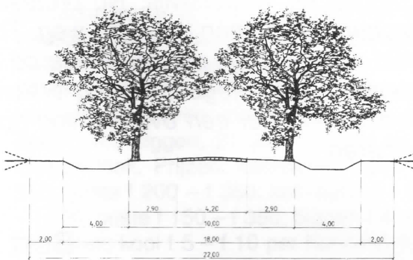
Fig. 1 het ideale profiel van de Rijksweg in het bestek van 1827
